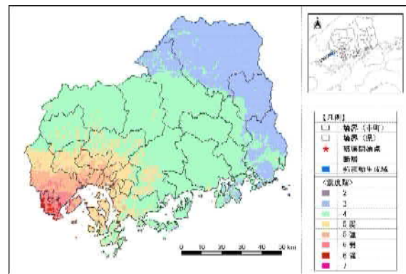
岩国－五日市断層帯（岩国断層区間）
