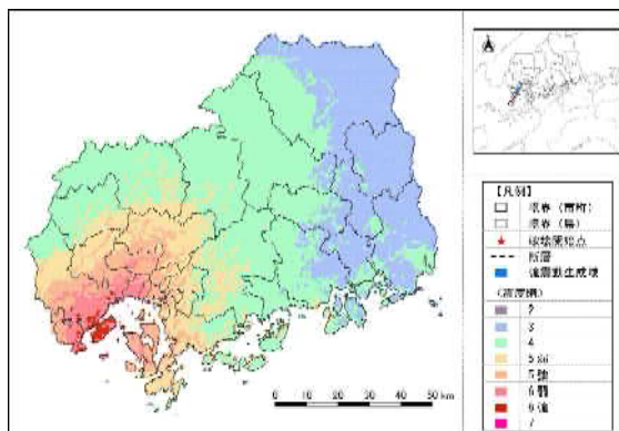
広島湾－岩国沖断層帯
