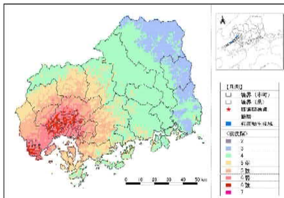
岩国－五日市断層帯（3 連動）
