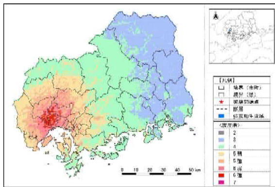
岩国－五日市断層帯（五日市断層区間）
